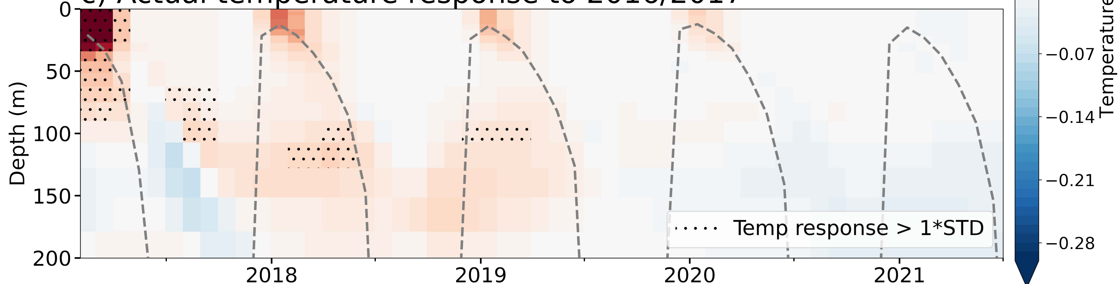
c) Actual temperature response to 2016/2017
